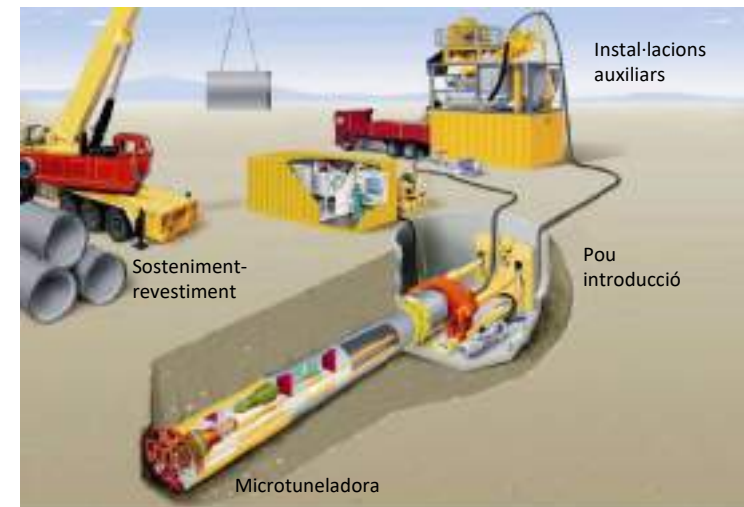
Microtuneladora i instal·lacions auxiliars
